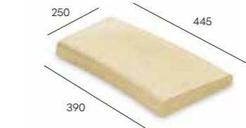
6 raio de curvatura 1500 curvature radius 1500 (445/390) x 250 x 30 - 50 mm bordadura côncava concave border
