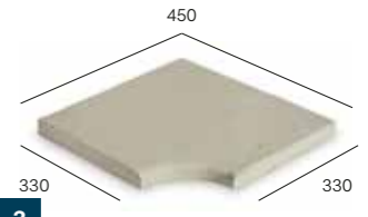
3 450 x 330 x 40 mm canto interno raio 150 radius 150 internal corner
