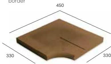
4 977/7 450 x 450 x 40 mm canto interno raio 150 radius 150 internal corner
